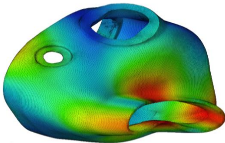
応力解析 (応力集中箇所の調査)
